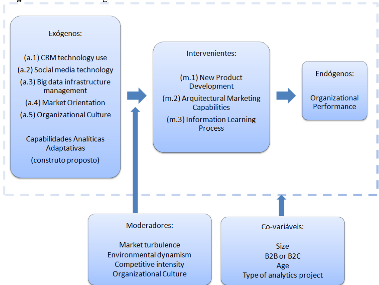
Figura 4 - Rede nomológica
