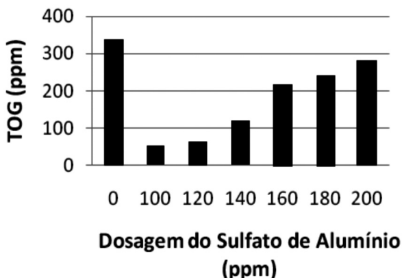
Gráfico 2: TOG versus sulfato de alumínio
