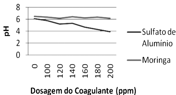
Gráfico 4: pH versus dosagem do coagulante
